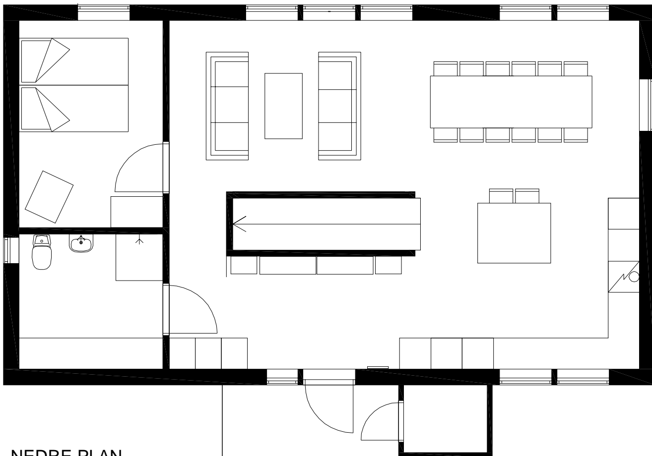
NEDRE PLAN
